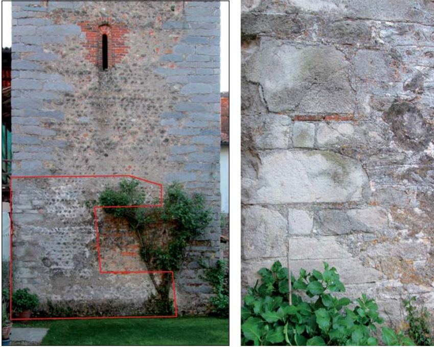
Fig. 10 - Massazza. 10.a. Il prospetto Nord-Est della parte basale della torre; in evidenza la porzione di muratura più antica; 10.b. Dettaglio del cantonale Est (foto G. Ardizio).
