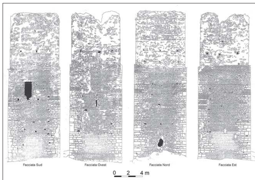
Fig. 6 - Rilievo architettonico dei prospetti esterni della torre delle Castelle a Gattinara (da FERRETTI, REFFO 1990, pp. 76-77).
