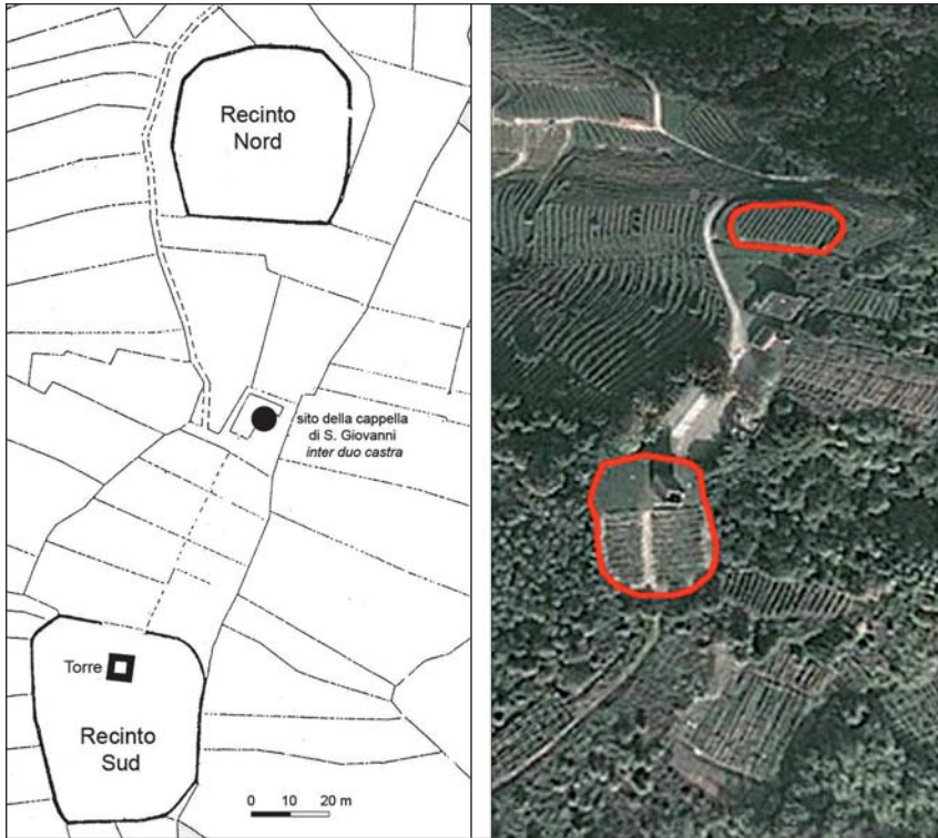
Fig. 5 - Gattinara. Il complesso delle Castelle: 5.a. Posizionamento delle emergenze architettoniche; 5.b. Veduta aerea del sito da Sud-Est (elaborazione di immagini fornite dall'Ufficio Tecnico del Comune di Gattinara).
