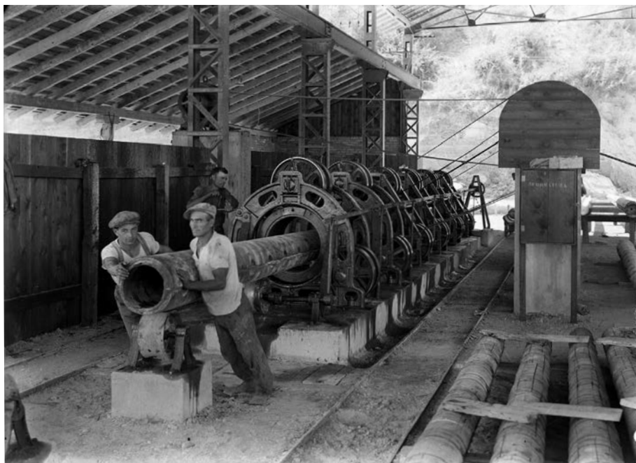
■ Rodolfo Rensi, Operai in un capannone durante la sformatura di un tubo , 1945-1965, gelatina ai sali d'argento su vetro. Archivio Studio Rensi, M_210260
