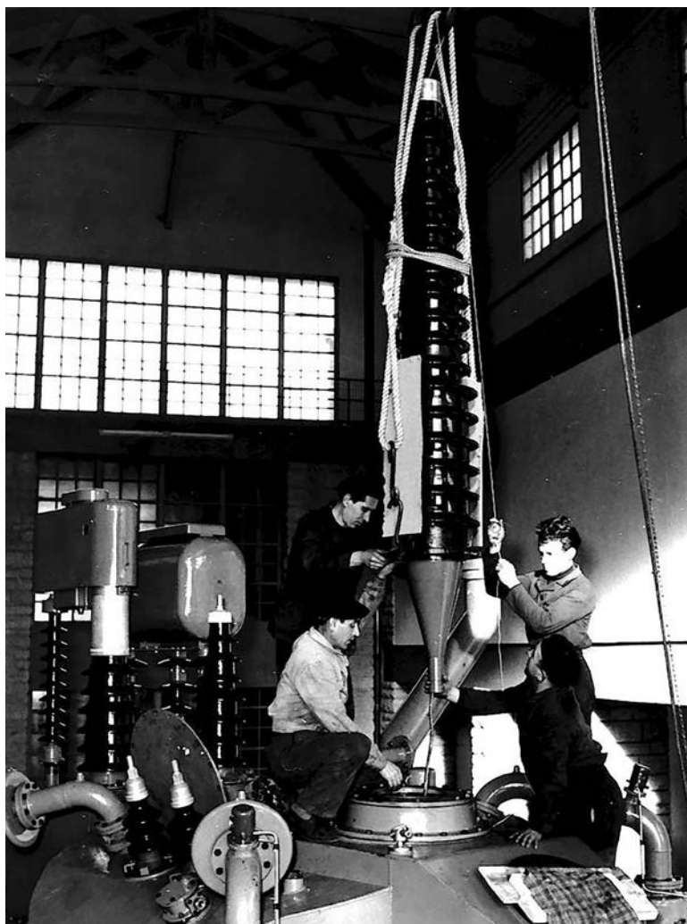
■ Fratelli Pedrotti (attr.), Vallelaghi, assemblaggio degli isolatori passanti di un trasformatore nella centrale idroelettrica di Santa Massenza, 1952-1960, gelatina ai sali d'argento su carta. Archivio del Servizio Energia. Provincia autonoma di Trento, M_198742
