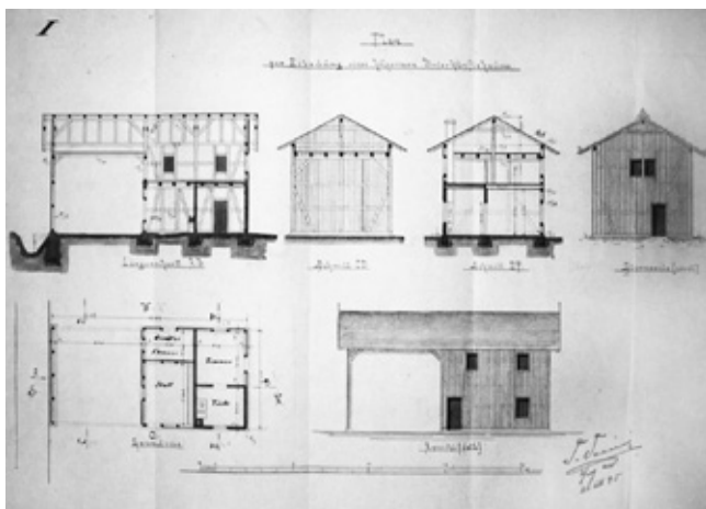
Figg. 1 e 2. APTN, ACARITRO, CARIRO, 09.0233, 1-2. Unterkunftsbaus (Bronzolo 1894). Progetti con diverse tecniche costruttive: Fachwerkswände (case a graticcio).
